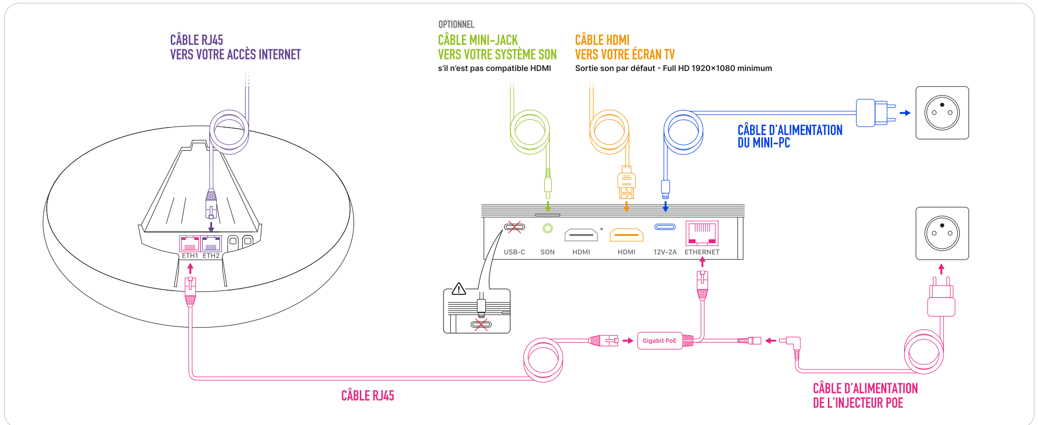
Raccordement mini-jack vers votre système son OPTIONNEL
