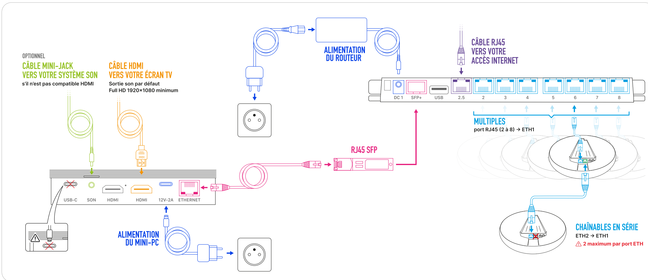
Raccordement mini-jack vers votre système son OPTIONNEL
